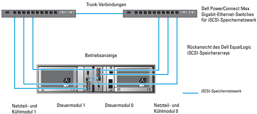
Abbildung 5-1. Empfohlene Netzwerkkonfiguration
