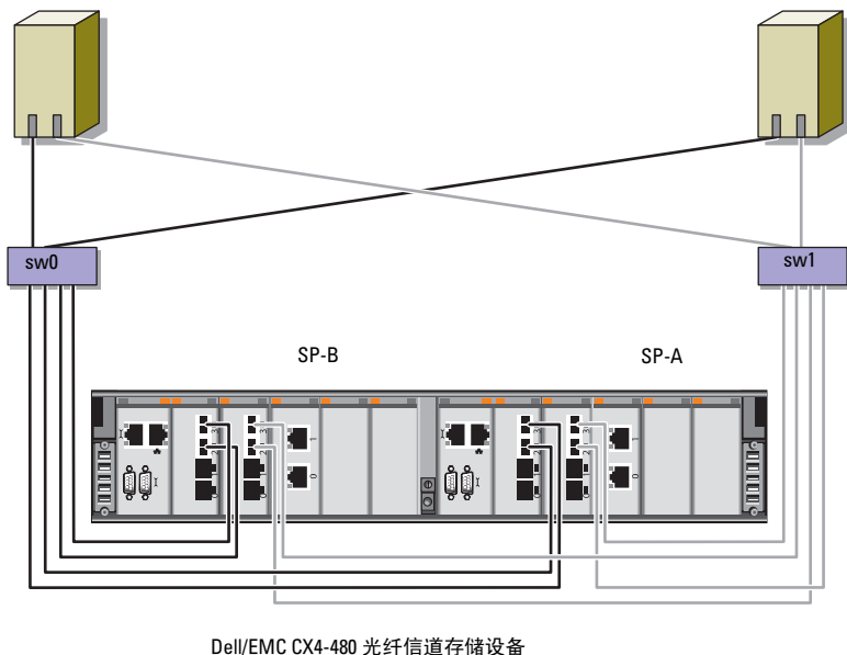
Dell/EMC CX4-480 光纤信道存储设备
