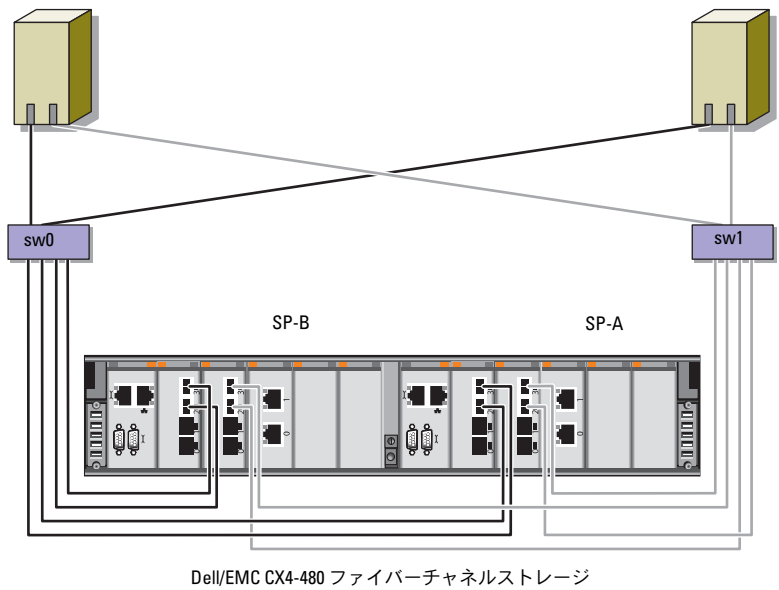
図 2-2. SAN 接続の Dell/EMC ファイバーチャネルクラスタのケーブル接続
